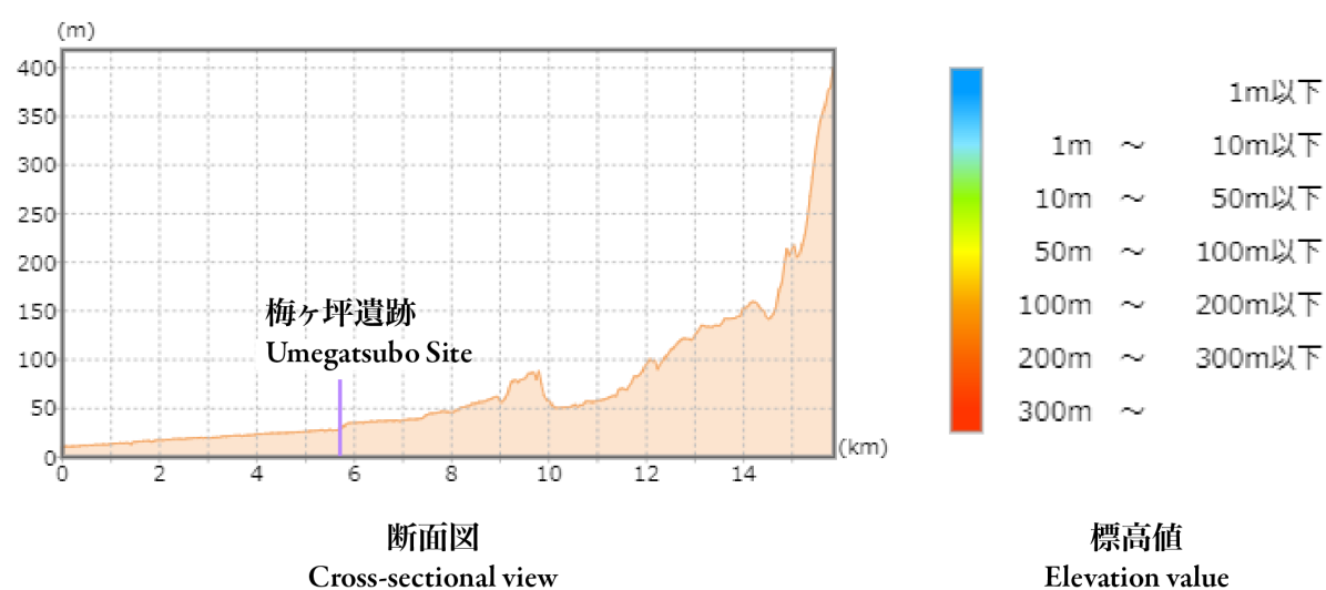
図 2： 標高図 Fig. 2: Elevation map
